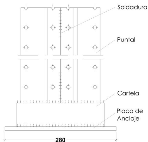
Alzado
