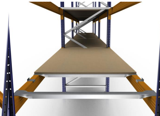
Nivel Picking con largueros de altillo
