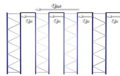
Estabilidad transversal
