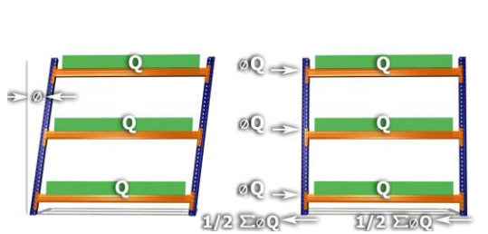
Estabilidad longitudinal
