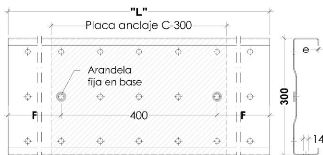
Alzado y perfil base doble 300
