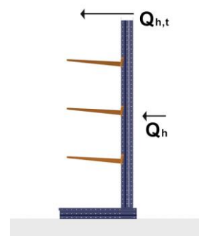
Estabilidad transversal
