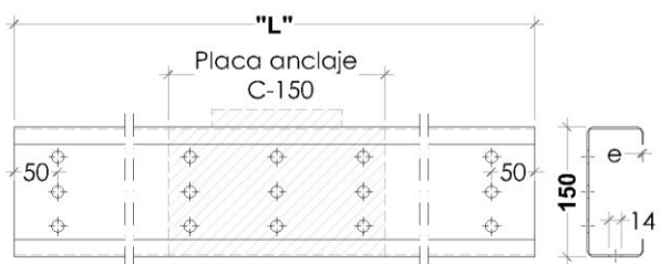
Alzado y perfil base doble 150
