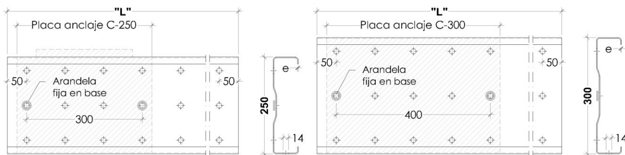
Alzado y perfil base simple 250 (Izq/Der)
