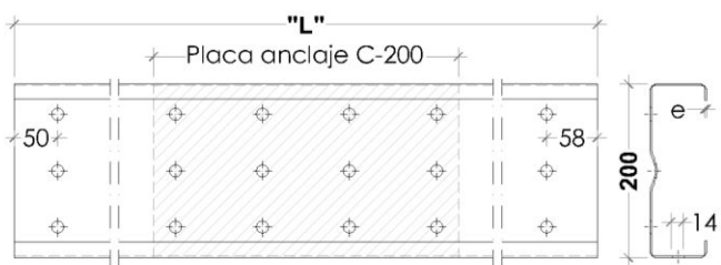
Alzado y perfil base doble 200
