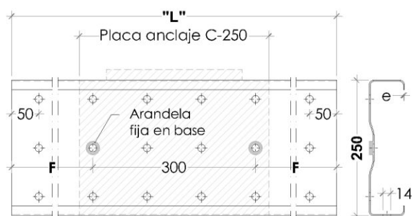
Alzado y perfil base doble 250
