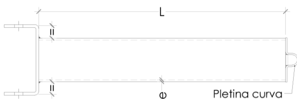
Planta
