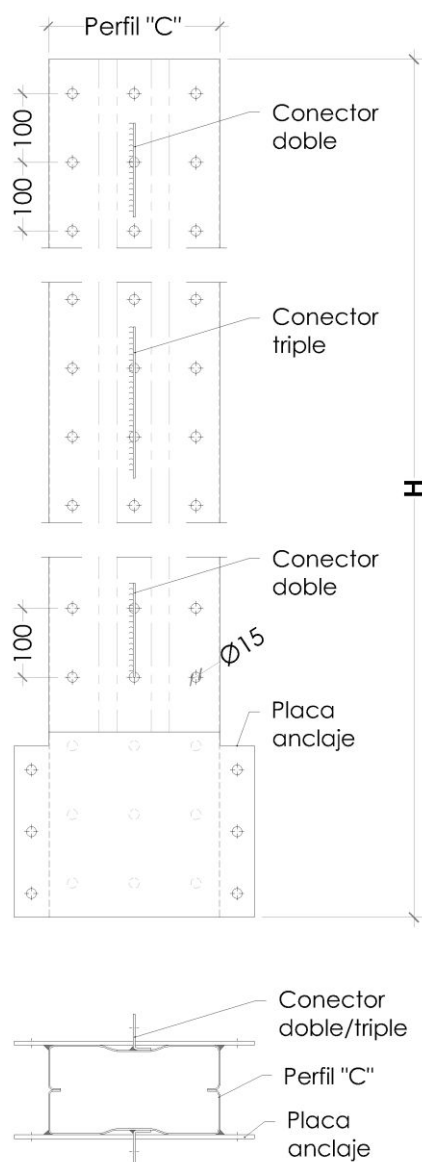
Planta y alzado genérico columna
