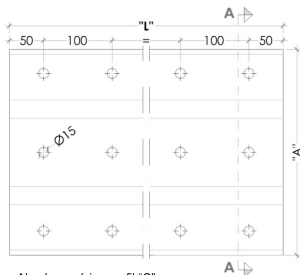
Alzado genérico perfil "C" L = corte de perfil
