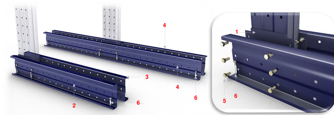
Esquema bases simples, dobles y detalle de fijación a columna
