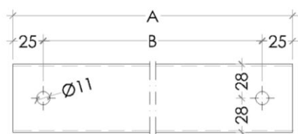
Alzado transversal
