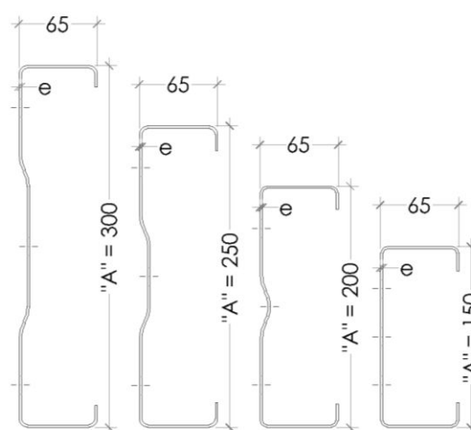
Sección A-A perfiles "C" e = 2, 2.5, 3 ó 4 mm
