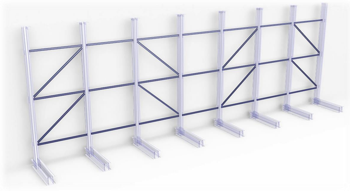
Esquema estándar de posicionamiento de diagonales y transversales
