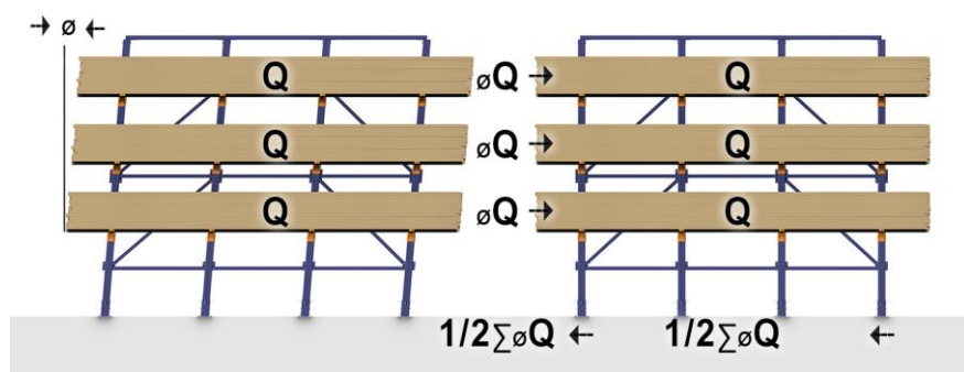
Estabilidad longitudinal
