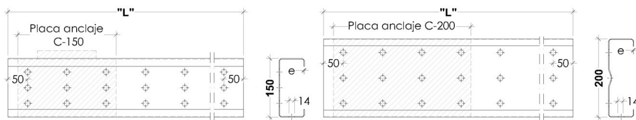
Alzado y perfil base simple 150 (Izq/Der)
